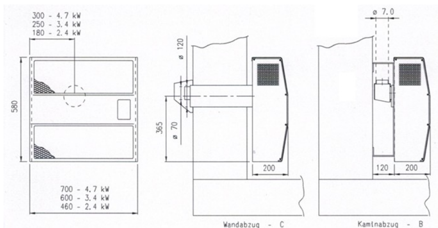
Masse T—Serie (** Kaminausführung nur noch auf Anfrage)
