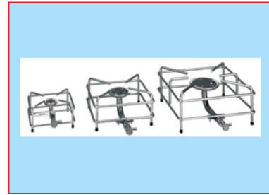
Nr. HK141173A / Nr. HK14117B / Nr. HK14117C Hockerkocher o. Zünds. 2,5kw, 6kw, 9,2kw nur Propan H12 B21 T27, H30 B30 T40, H40 B20 T50
