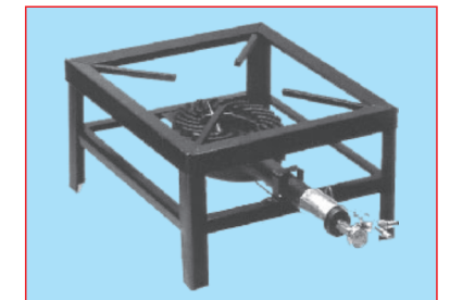
Nr. HK141179 Hockerkocher 9,2kw m. Zünds. nur Propan H25,5 B38 T38
